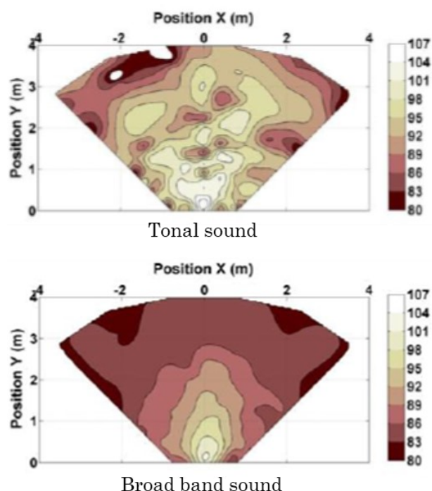
図2 “Tonal sound”及び”Broad band sound” 発音時の車両後方の音場 3)
