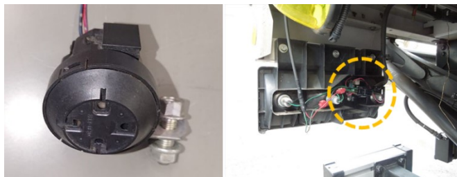
図 1 後退時警報装置とその取付け例
