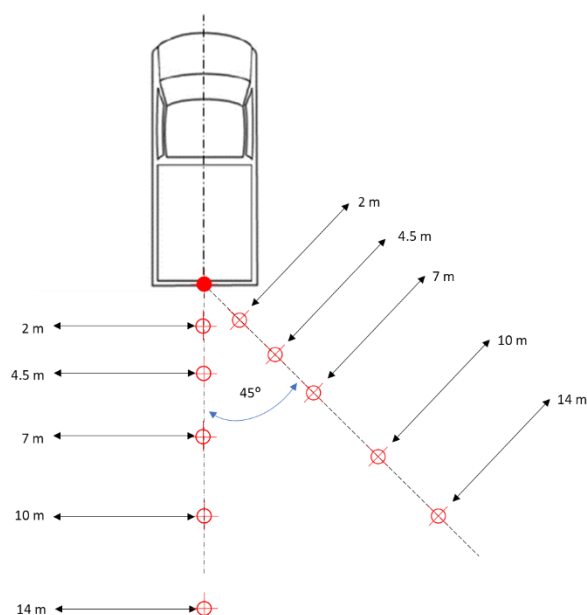
図3 車両装着時の試験法策定時に検討を行った 測定点のレイアウト
